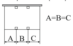
Схема расположения фиксаторов
